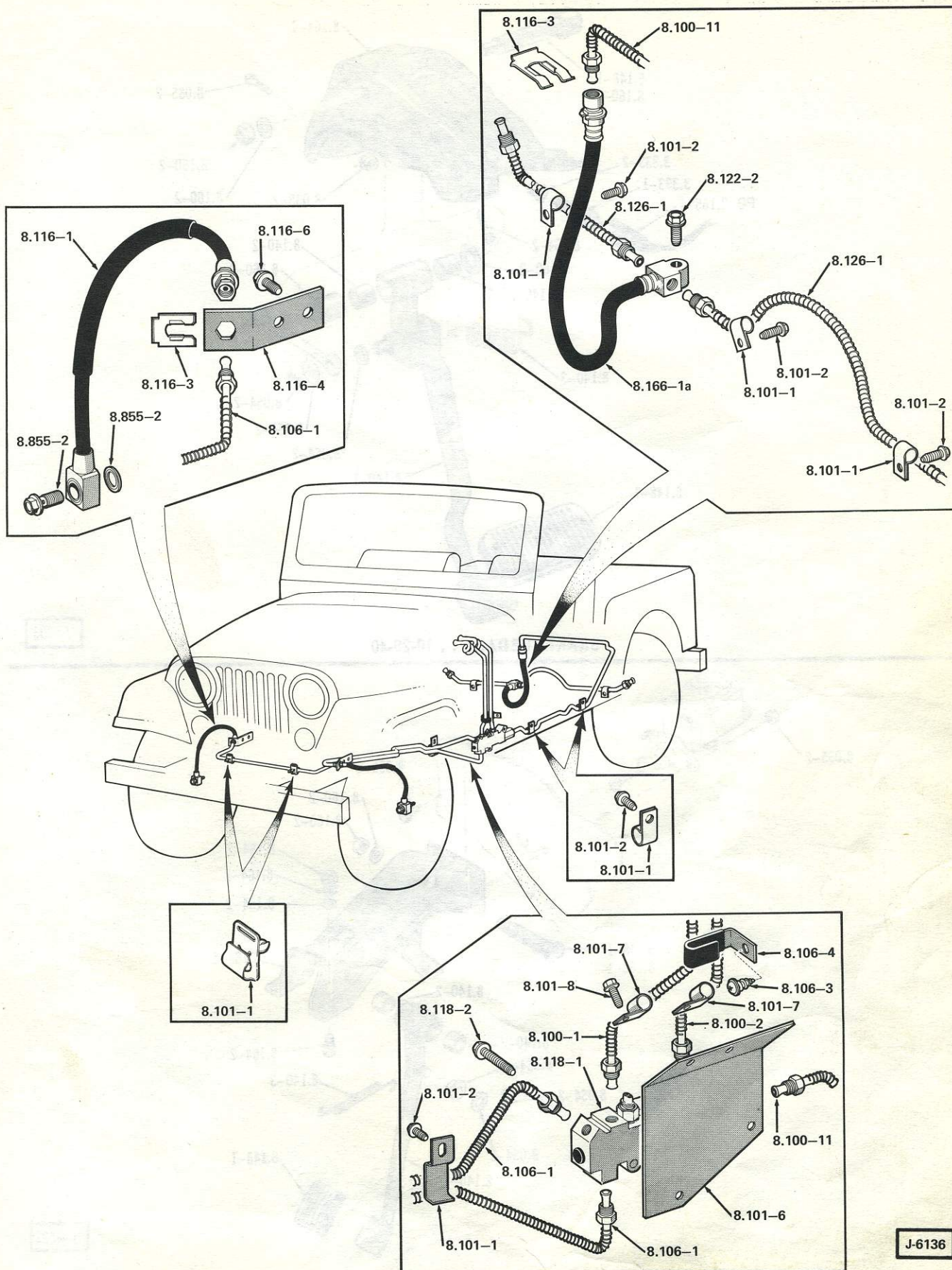
BRAKE LINES... 1977/ 80-90 (WDB)
