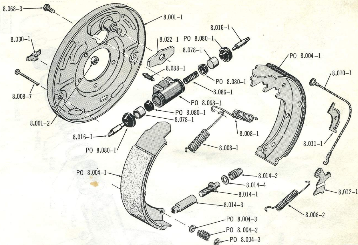
FRONT BRAKE . . . 80-90 (LDB)
