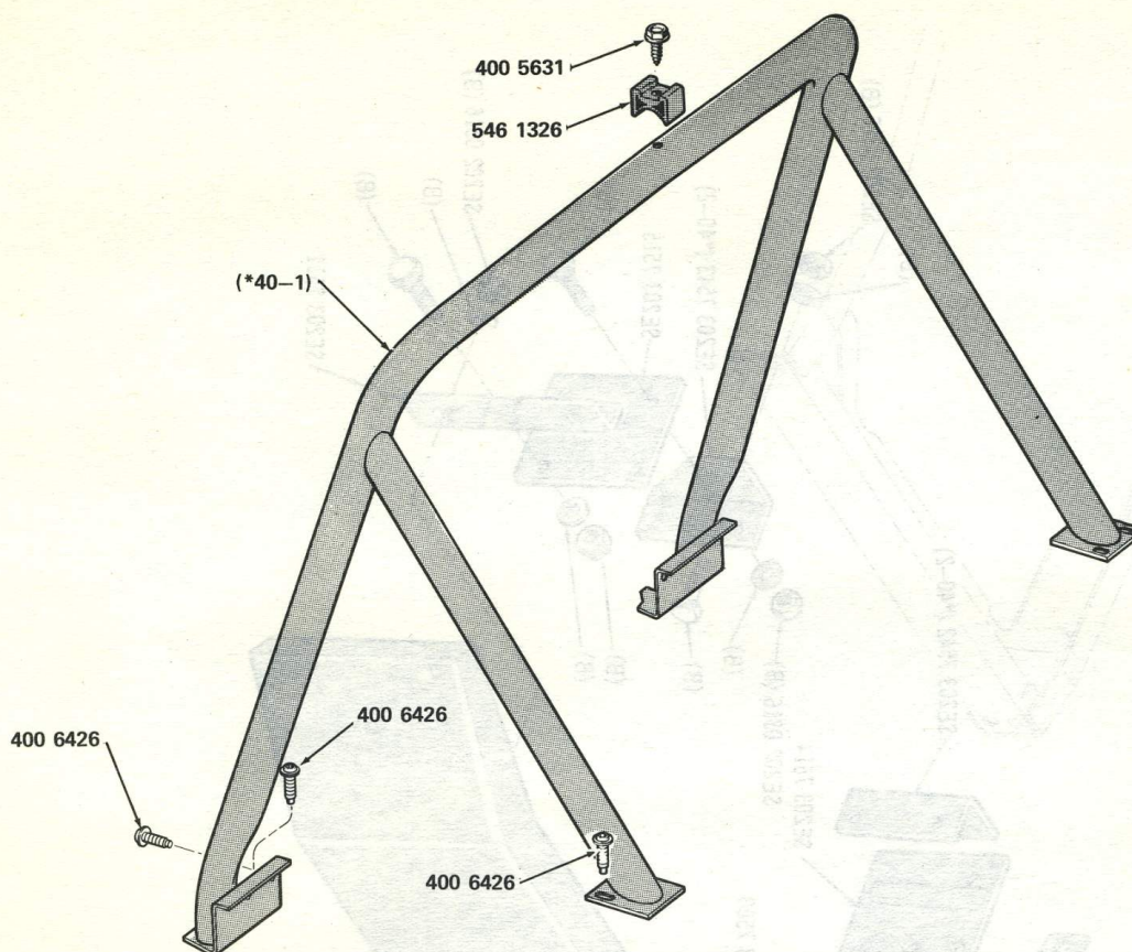
ROLL BAR . . . 83-93 (1979 - TYPE 2 , 1980)
